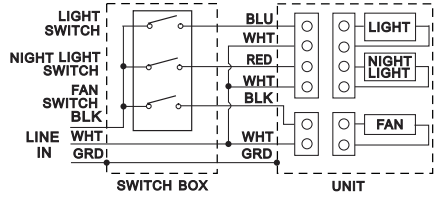
Fan with PCLK / PCLEDK
