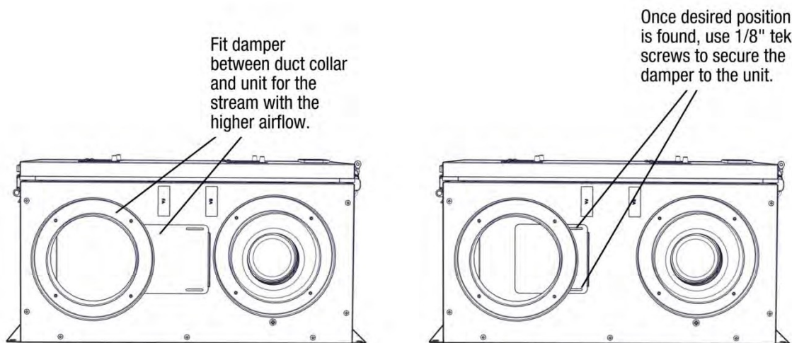
Installation du clapet
